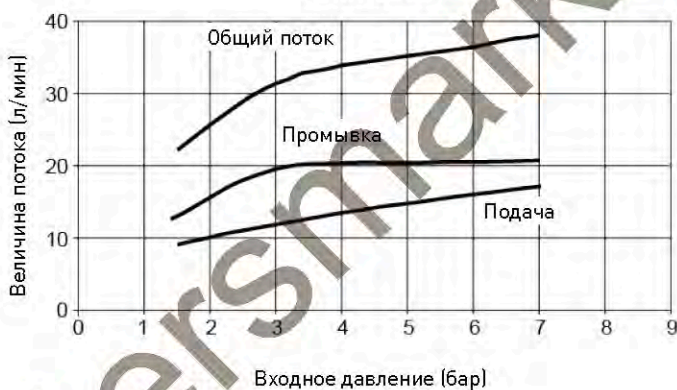
ИНЖЕКТОР 7
